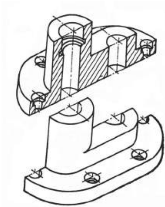
شكل ( 6-1 ) : المنظور بعد القطع
