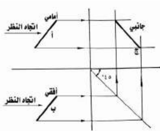
الشكل ( أ ) : استنتاج المسقط الجانبي للمستقيم المائل
