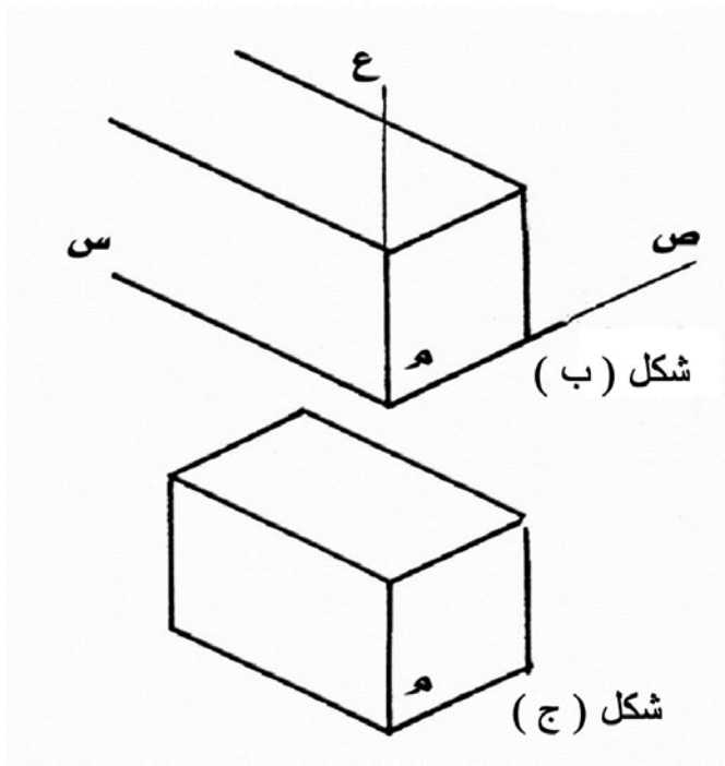
شكل ( 5-5 ) خطوات رسم المنظور المتوازي
